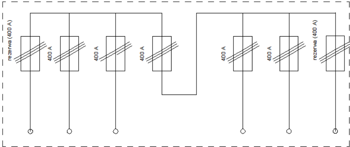
Rysunek nr 3. Złącze ZK - 22
