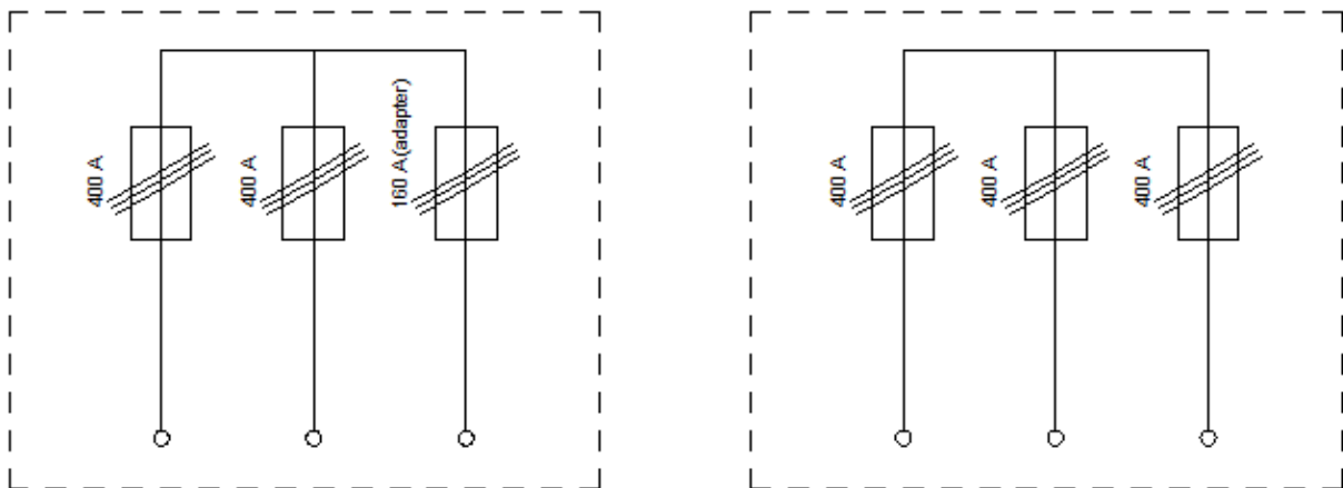
Rysunek nr 2. Złącze ZK - 2
