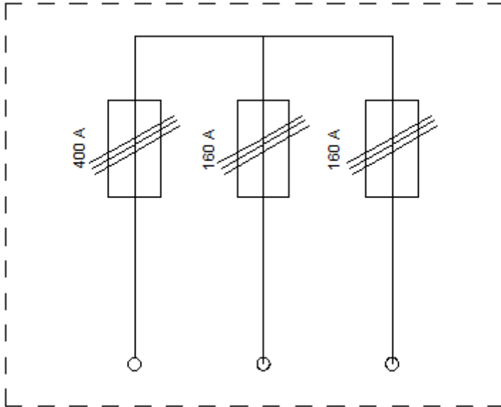
Rysunek nr 1. Złącze ZK – 1
