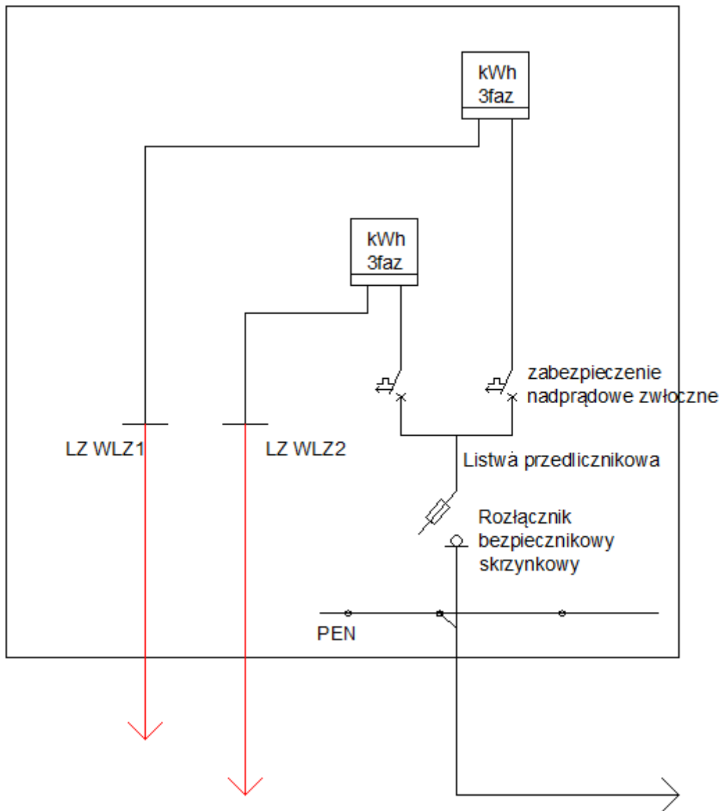
nr 1. Szafka wolnostojąca SP – 2
