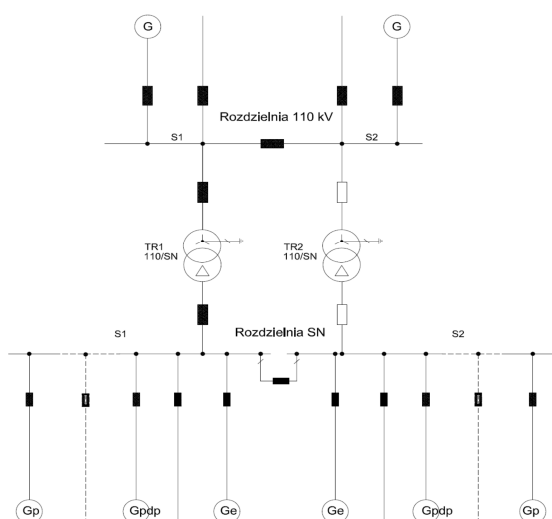
Konfiguracja maksymalna stacji 110/SN
