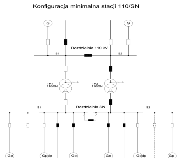
Rys.2. Konfiguracja minimalna GPZ/RPZ
